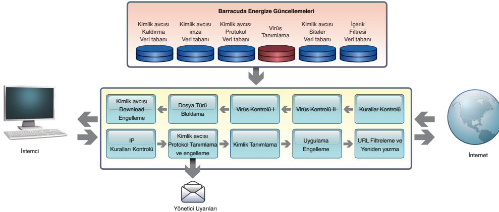
Barracuda Web Filter Altyapısı
